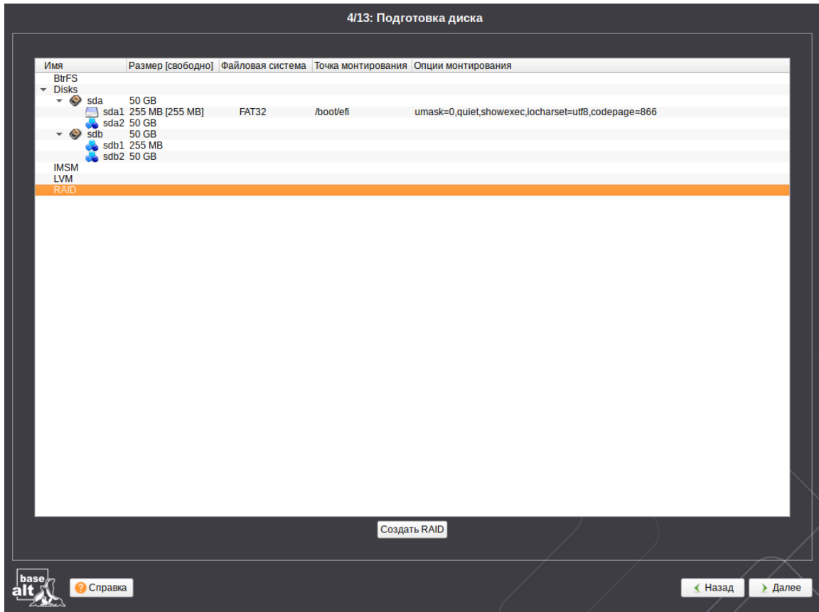
Рис. 12 Установка. Выбор типа RAID-массива
